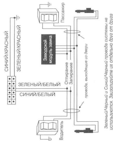
Схема 1. 3-проводная система центрального замка, управляемая сигналом отрицательной полярности (большинство автомобилей японского производства)
