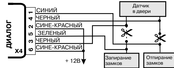
Рис. 9. Схема подключения к блоку центрального замка с управлением импульсами со сменой полярности
