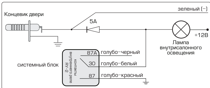
Схема подключения внутрисалонного освещения с отрицательной полярностью
