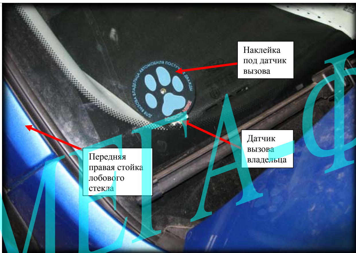
Рис. 8: Возможное место установки датчика вызова владельца.
