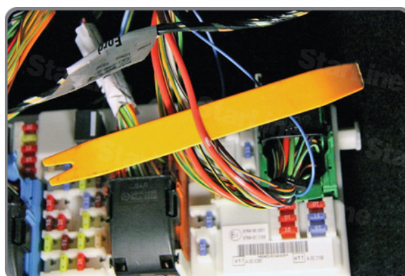
Фото 11.4. Постоянный плюс (красный)
