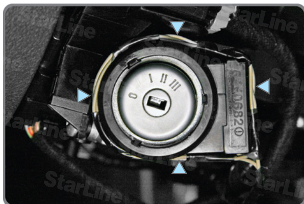
Фото 9. Обход штатного иммобилайзера
