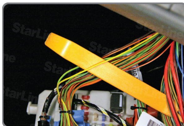
Фото 11.2. Аксессуары (ACC-желтый)
