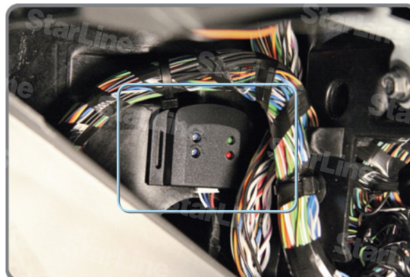
Фото 5.4. Датчик удара
