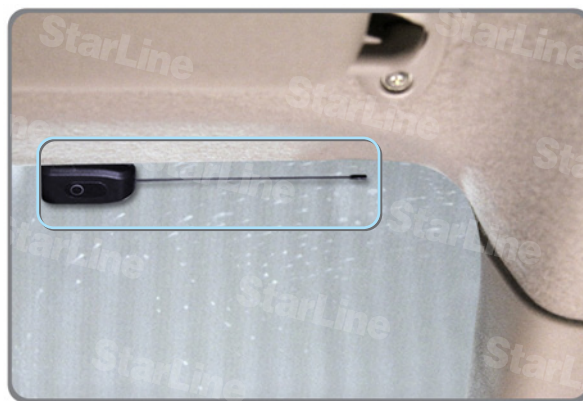
Фото 5.2. Антенна на лобовом стекле
