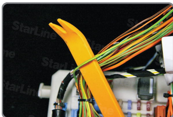
Фото 11.1. Зажигание (IGN-зеленый с желтой полосой)
