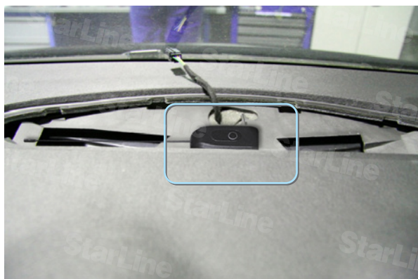
Фото 5.3. Антенный модуль
