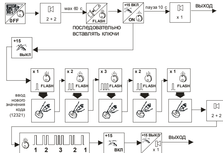
Рис.8.10. Программирование электронных ключей и модификация персонального кода при первом включении напряжения питания.
