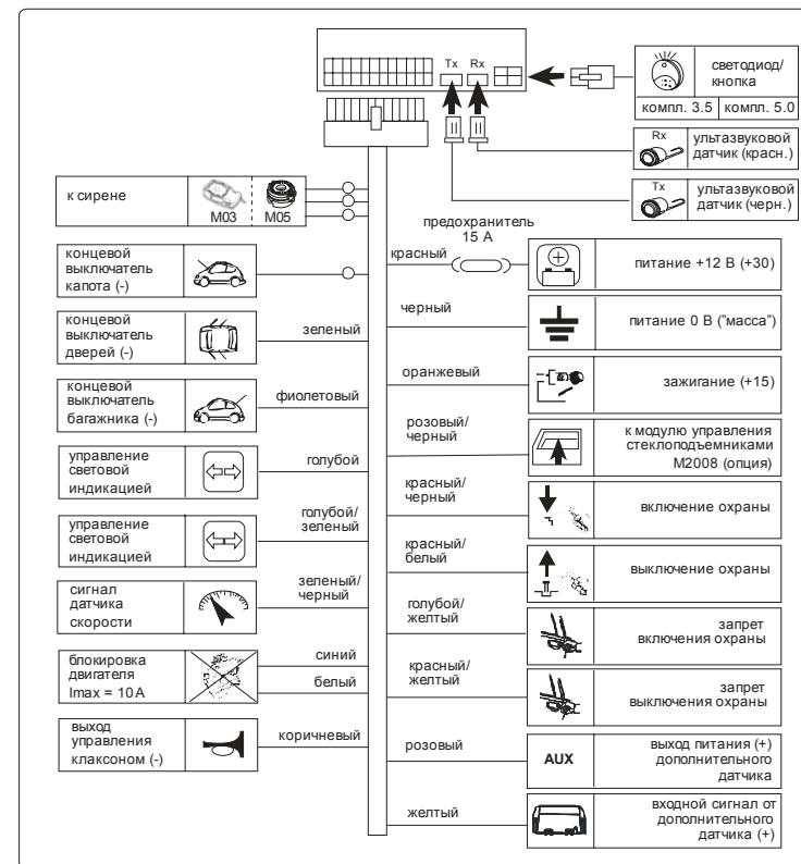
Рис.9.1. Схема подключения системы HPB TOP PLIP .
