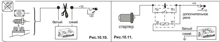
Рис.10.10, 10.11. Варианты блокировки запуска двигателя.
