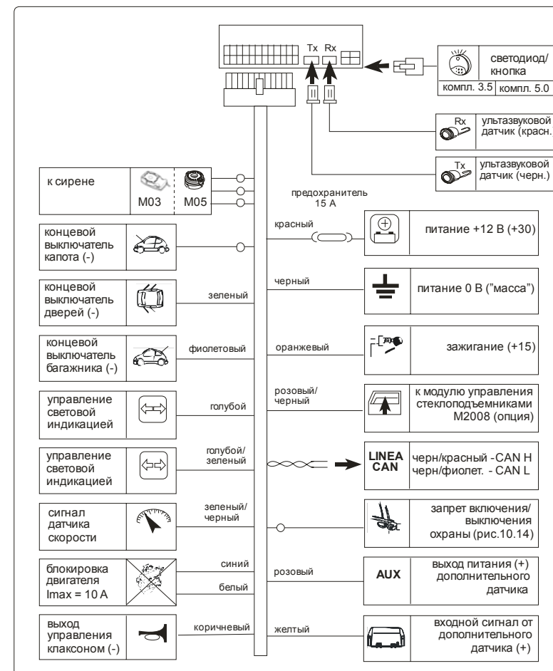
Рис.9.1. Схема подключения системы HPB VW CAN .
