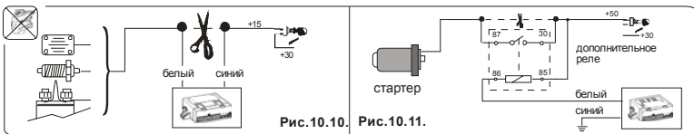
Рис.10.10, 10.11. Варианты блокировки запуска двигателя.
