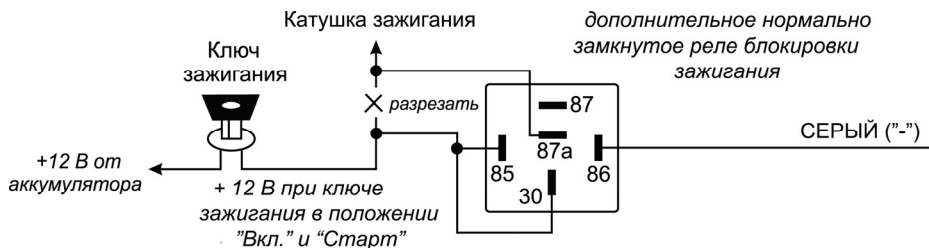
Схема подключения СЕРОВОГО провода для блокировки цепи зажигания автомобиля:
