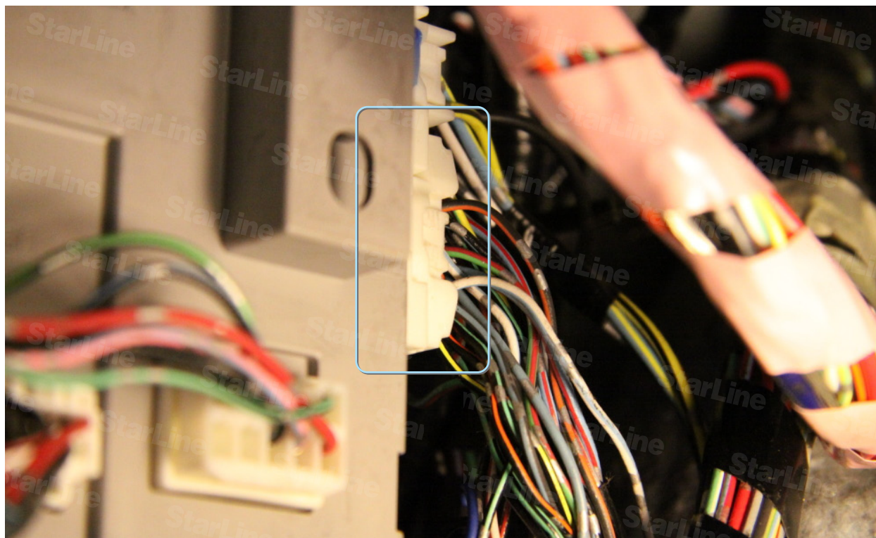
Фото 10.2. Разъем «1» блока BCM
