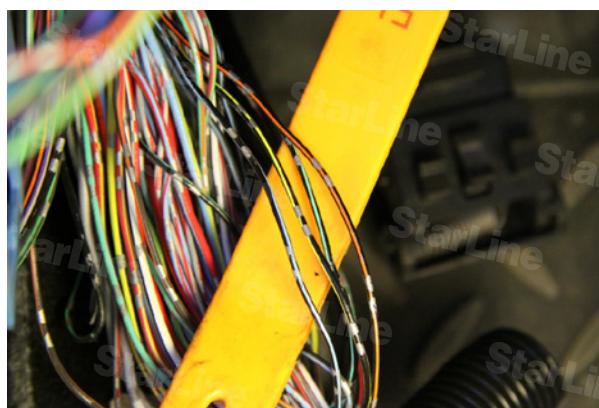
Фото 9.1. Концевики дверей (черно-желтый, черно-голубой, черно-салатовый, черно-оранжевый)
