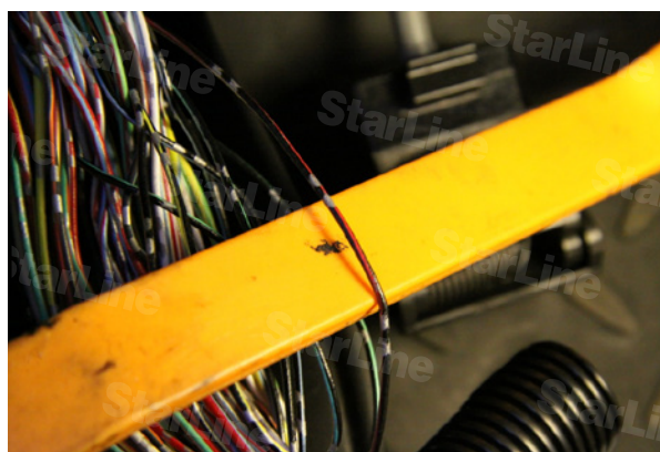
Фото 9.2. Концевик багажника (черно-красный)
