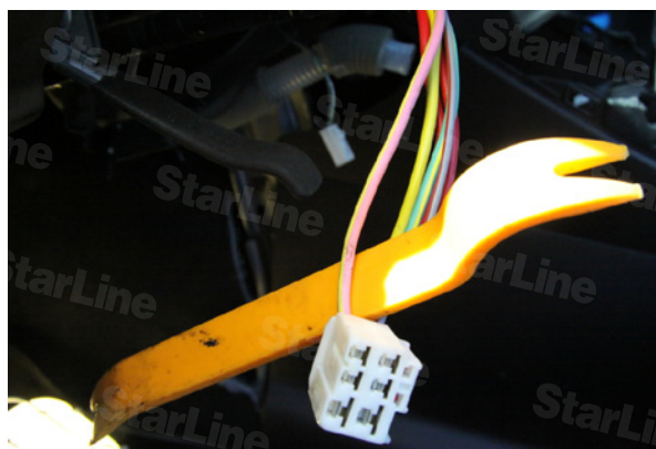
Фото 14.2. Зажигание2 (IGN2 розово-желтый)
