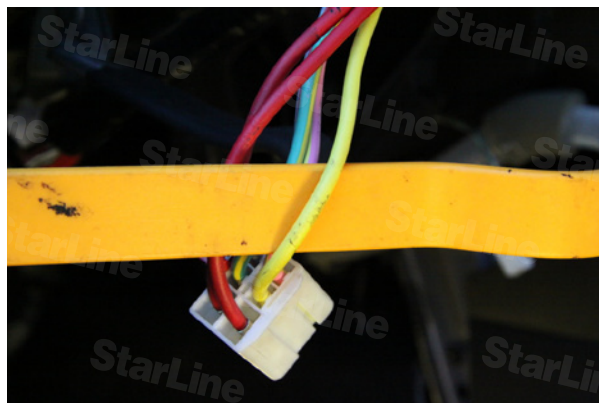
Фото 14.3. Аксессуары (АСС желтый)
