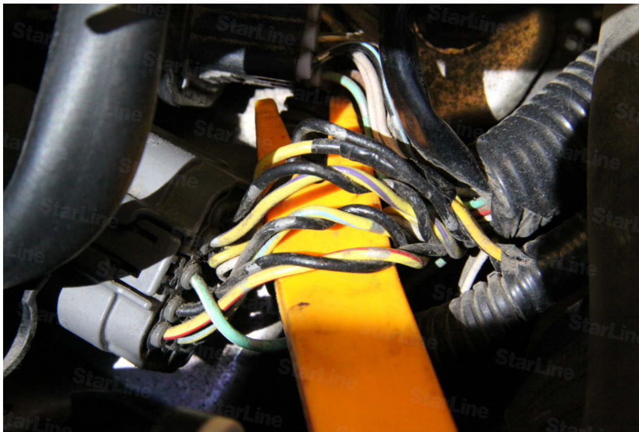
Фото 6.6. Контроль работы двигателя. Любой из желтых проводов в витых парах
