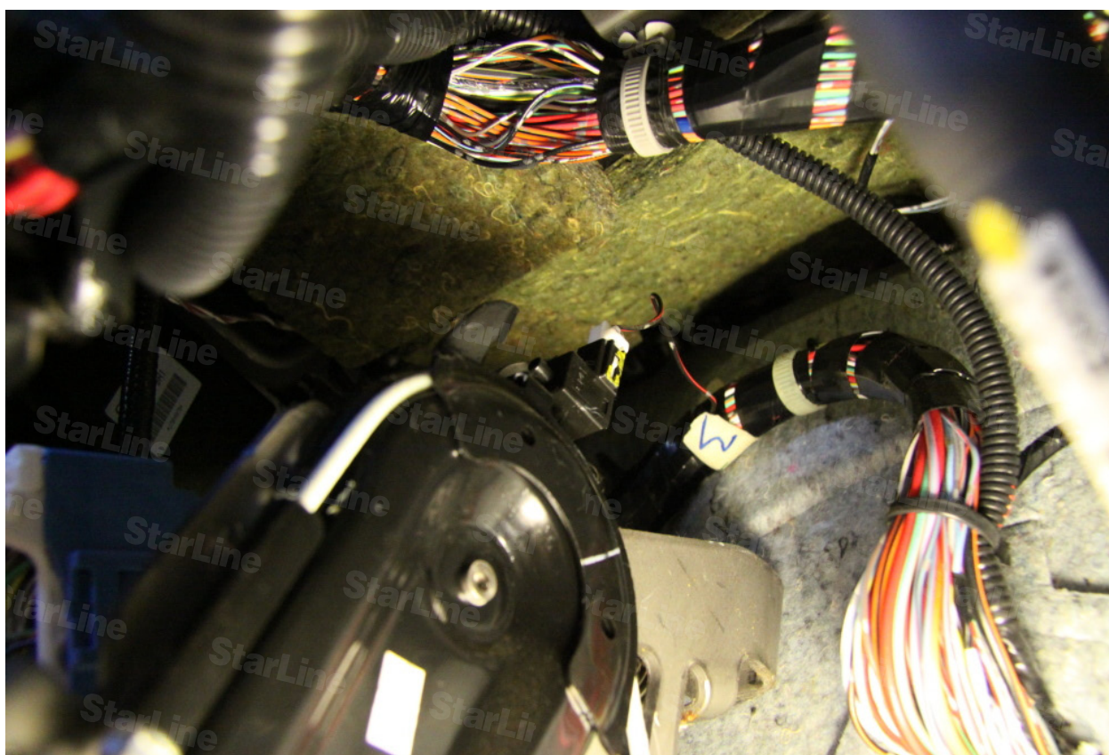
Фото 11. Разъем педали стояночного тормоза
