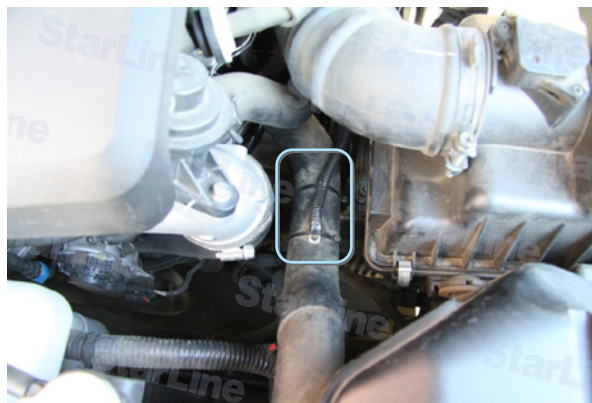
Фото 6.4. Датчик температуры. Крепление хомутами
