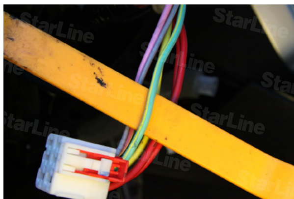
Фото 14.1. Зажигание1 (IGN1 зелено-желтый)
