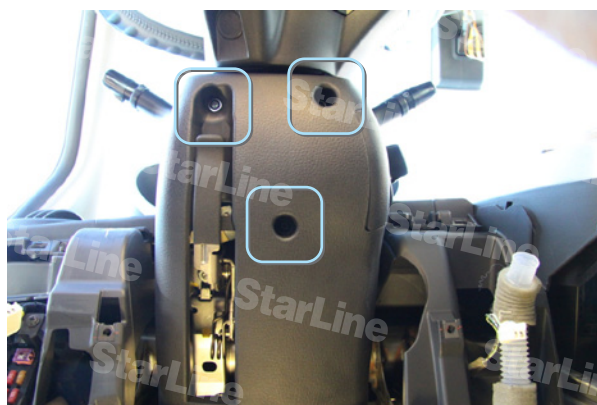
Фото 4.1. Крепление облицовки рулевого вала
