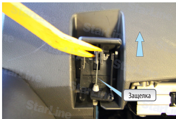
Фото 3.1. Рукоятка открытия капота
