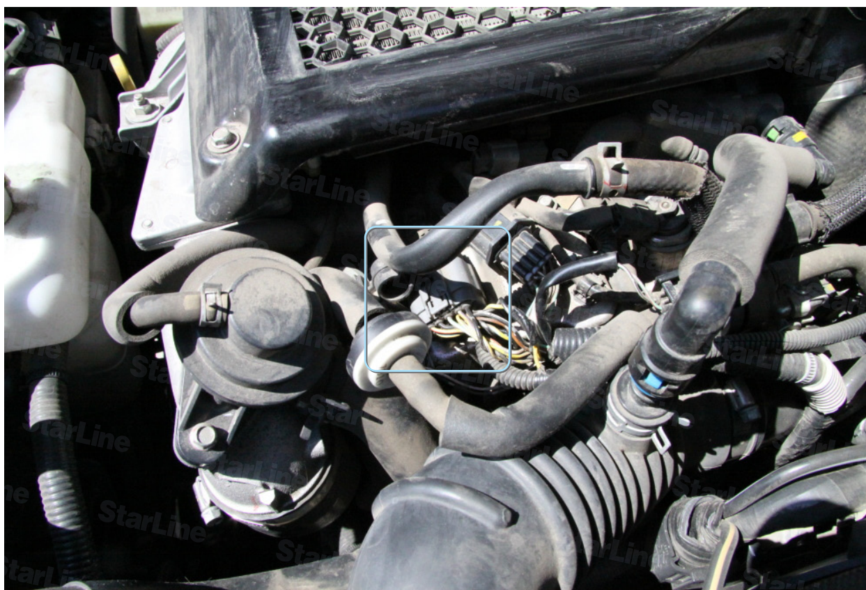
Фото 6.5. Разъем форсунок
