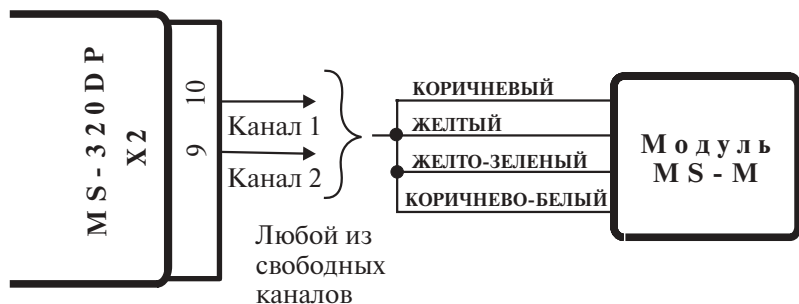
Рис. 11. Подключение модуля MS-M к автосигнализации MS-320DP для закрывания стекол при постановке на охрану
