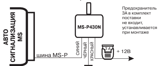
Рис. 1. Типовая схема подключения пейджера MS-P430N к автосигнализации MS по шине MS-P
