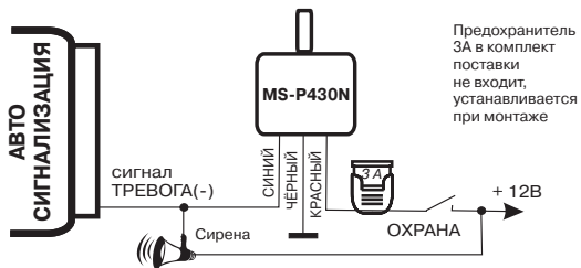
Рис. 3. Варианты схем подключения пейджера MS-P430N к обычной автосигнализации
