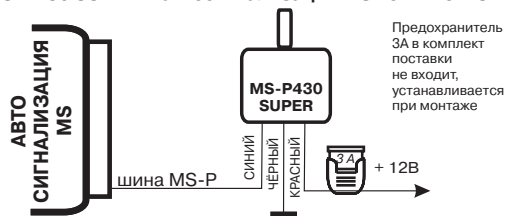
Рис. 1. Типовая схема подключения пейджера MS-P430 SUPER к автосигнализации MS по шине MS-P
