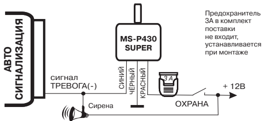
Рис. 3. Варианты схем подключения пейджера MS-P430 SUPER к обычной автосигнализации
