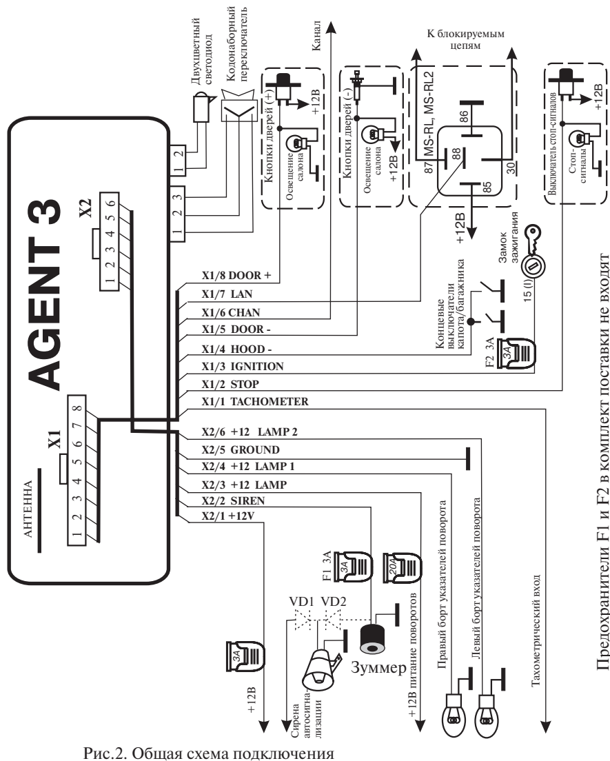
Рис.2. Общая схема подключения
