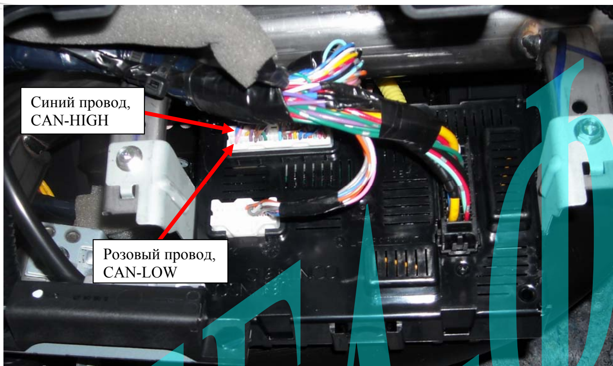
Рис. 1: Подключение к CAN шине автомобиля на модуле BCM.
