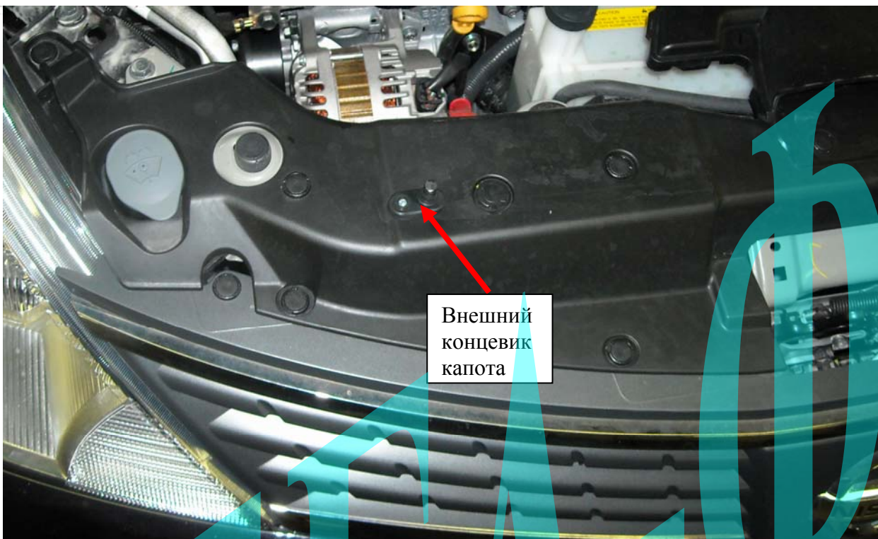
Рис. 6: Возможное место установки концевика капота.
