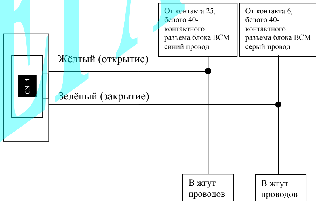
Схема 1: Подключение центрального замка.
