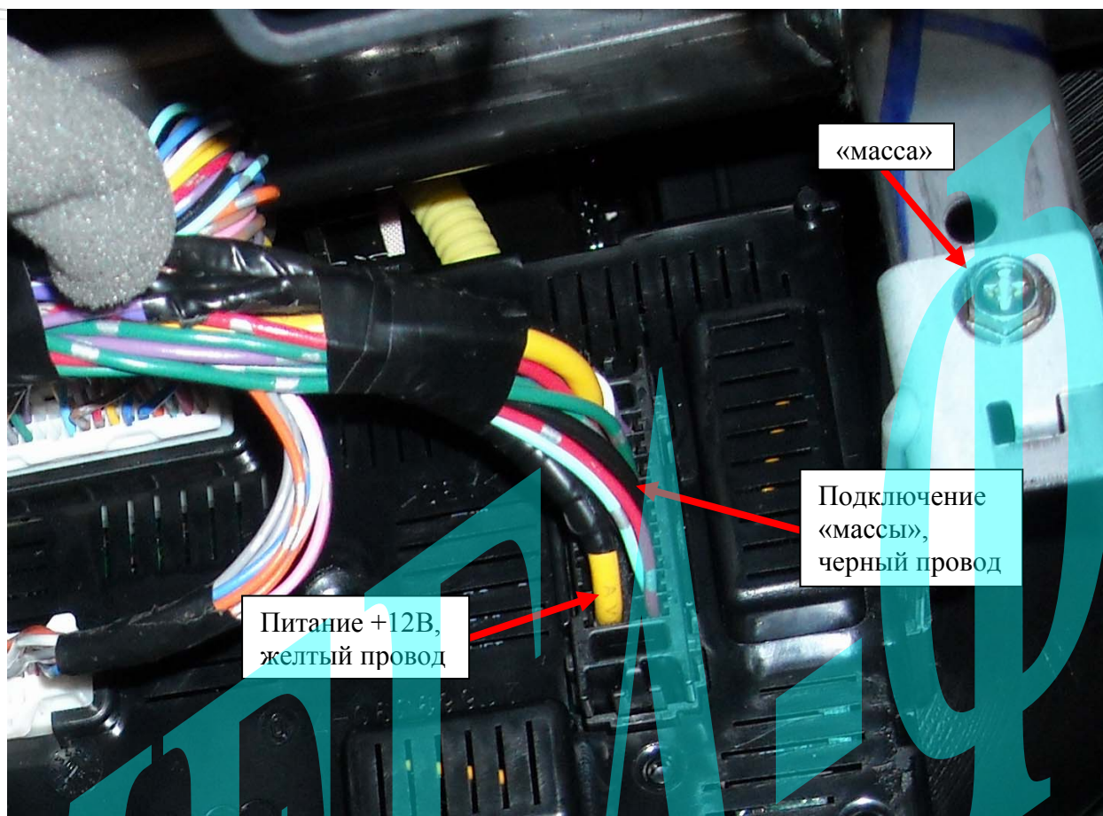
Рис. 12: Подключение питания и «массы».
