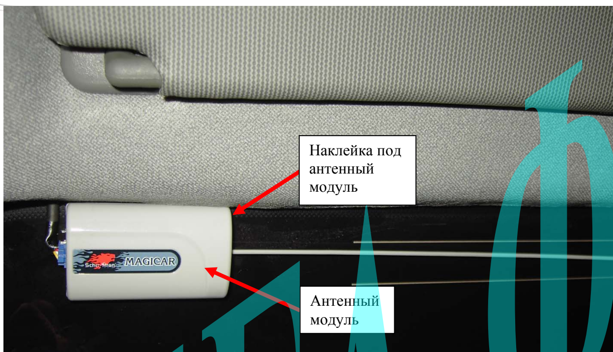
Рис. 12а: Антенный модуль системы Scher-Khan Magicar 5.
