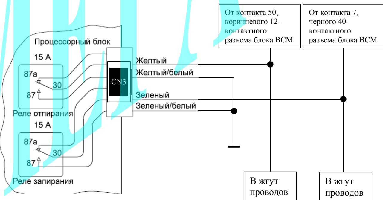
Схема 1: Подключение центрального замка.
