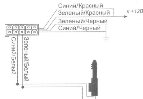
Схема 6. Установка дополнительных электроприводов
