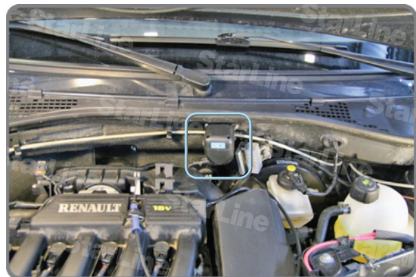
Фото 6.2. Общий вид
