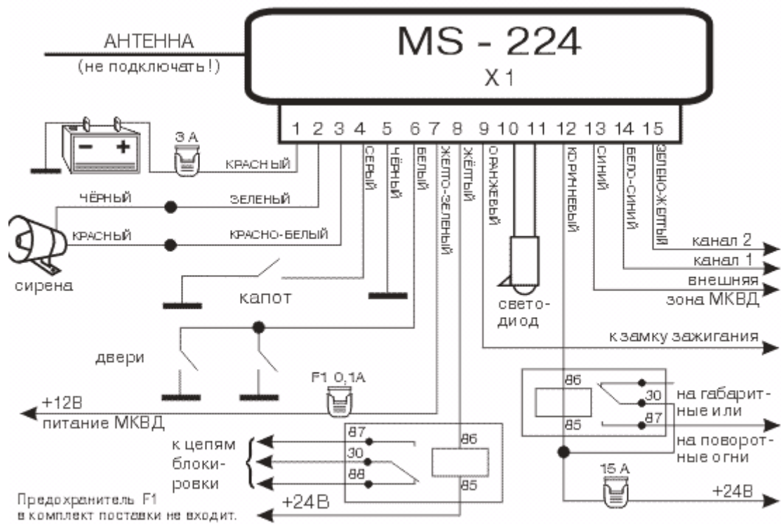
Рис. 2. Общая схема подключения
