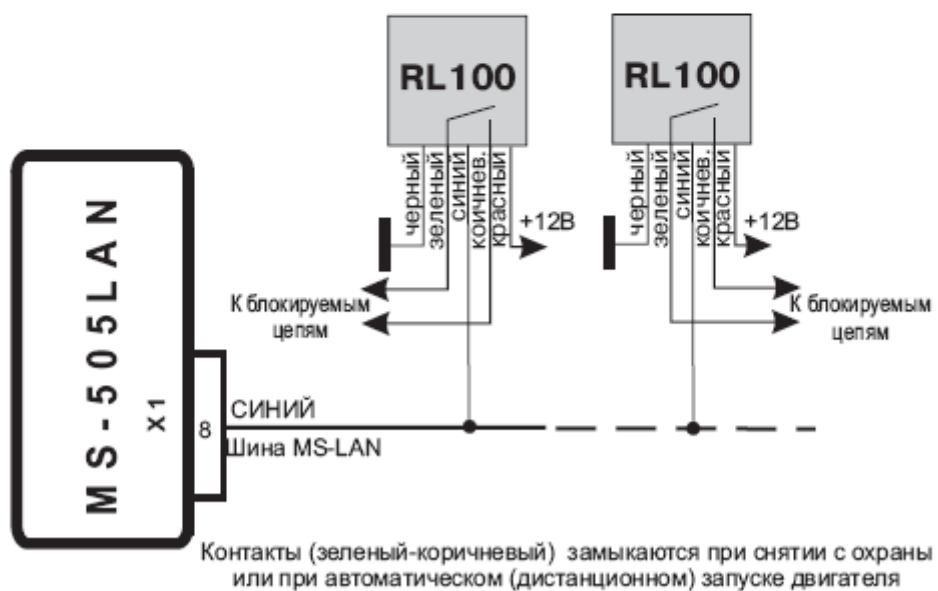
Рис.2. Схема совместной работы автосигнализации MS-505 LAN и реле блокировки RL100
