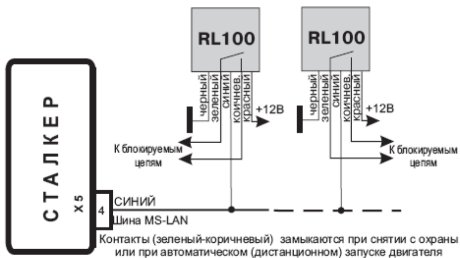
Рис.1. Схема совместной работы автомобильного охранного комплекса СТАЛКЕР и реле блокировки RL100
