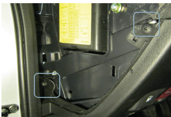
Фото 1.1. Снятие накладки торпеды, саморез и гайка
