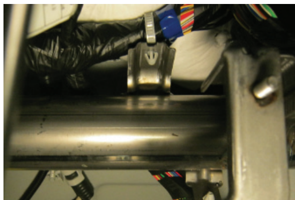
Фото 5.2. Крепление блока за поперечной балкой
