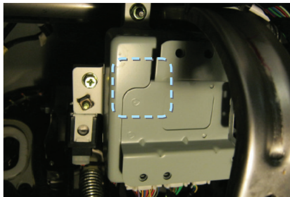
Фото 1.4. Место расположения блока управления центральным замком
