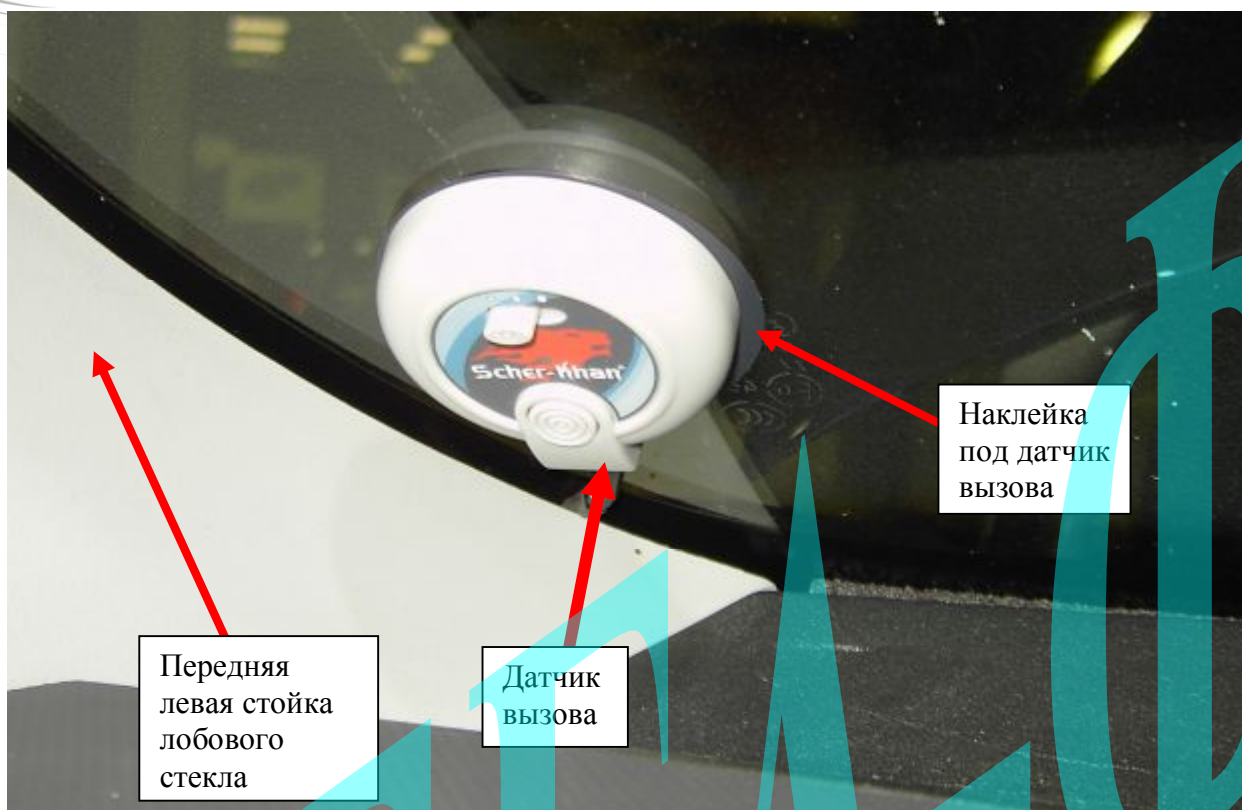
Рис. 7: Возможное место установки датчика вызова владельца.
