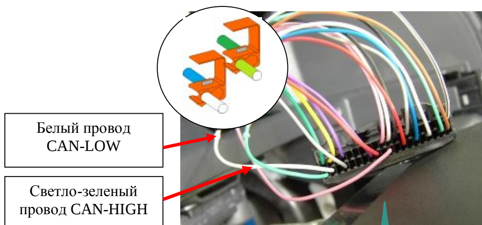
Рис.1: Подключение CAN шины на щитке приборов.
