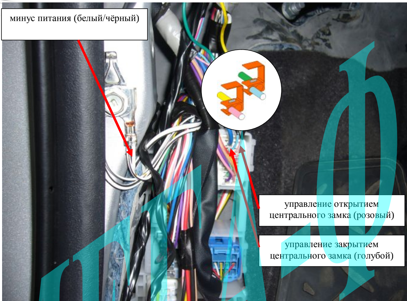
Рис. 1: Подключение управления центральным замком и минуса питания в левой кикпанеле.
