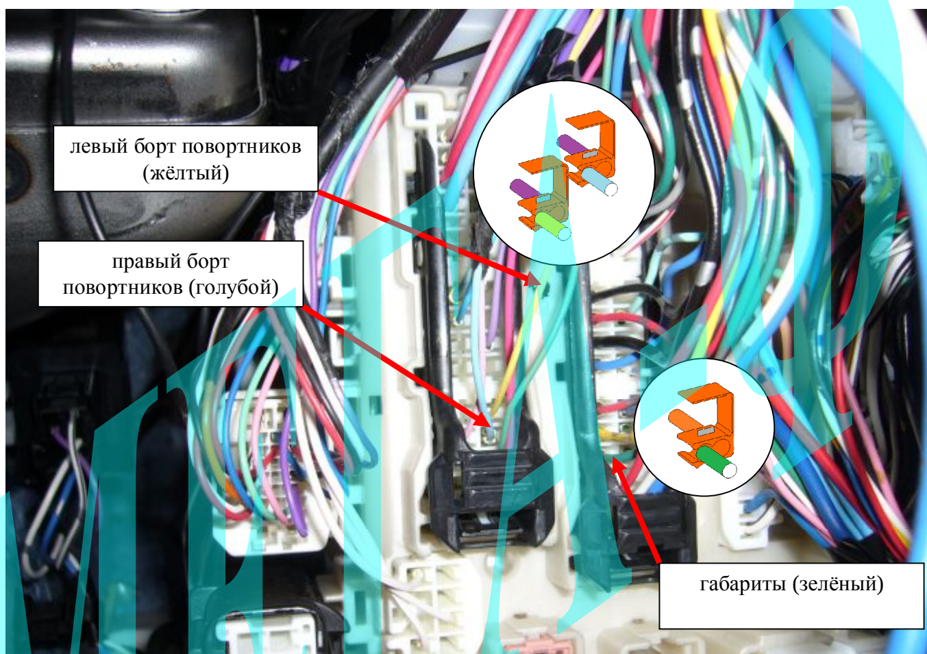
Рис. 2: Подключение аварийной сигнализации и контроля габаритных огней на монтажном блоке (слева от руля).
