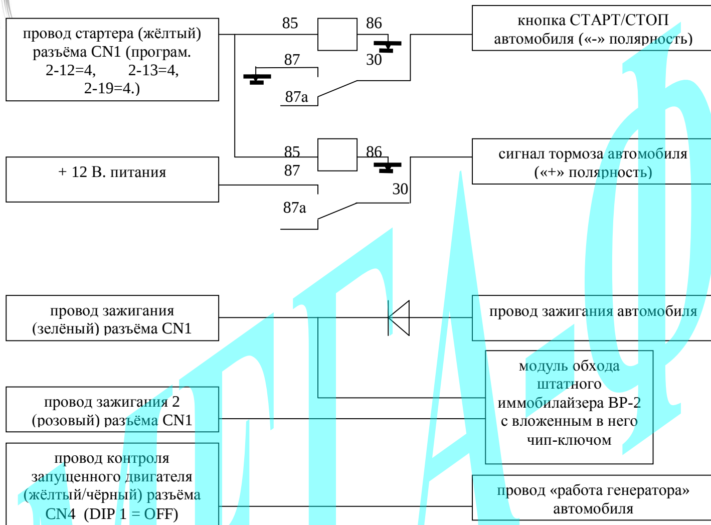
Схема 2: Реализация автозапуска.
