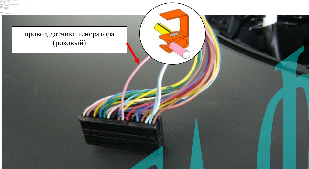
Рис.7: Подключение датчика генератора на разъёме комбинации приборов.
