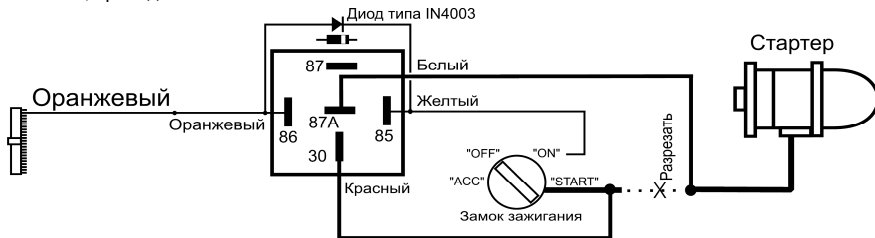
Цепь блокировки стартера
