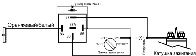
Цепь блокировки зажигания
