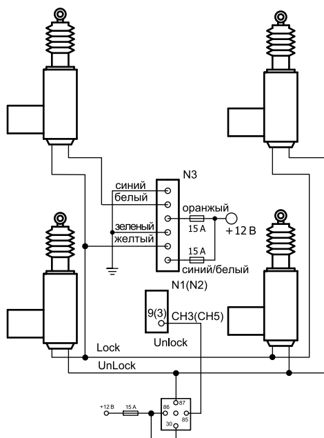
Схема управления электроприводами замков дверей при пошаговом (раздельном) отпирании водительской и пассажирских дверей автомобиля
